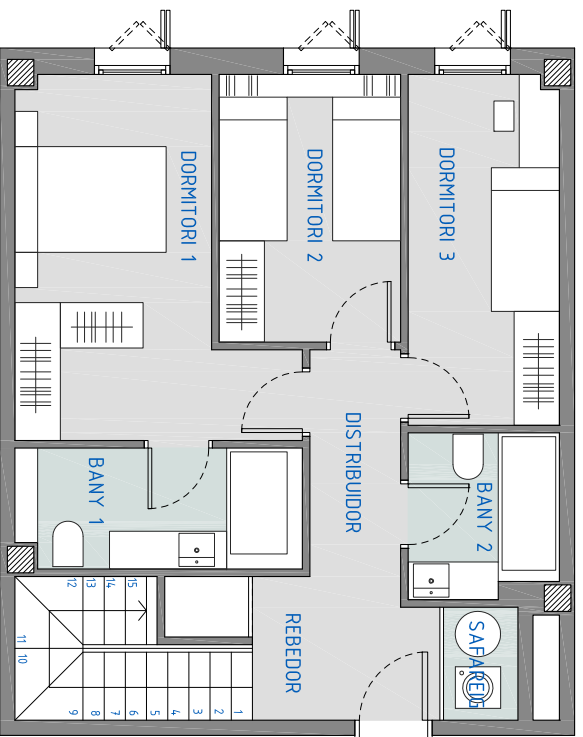
PLANTA SEGONA
