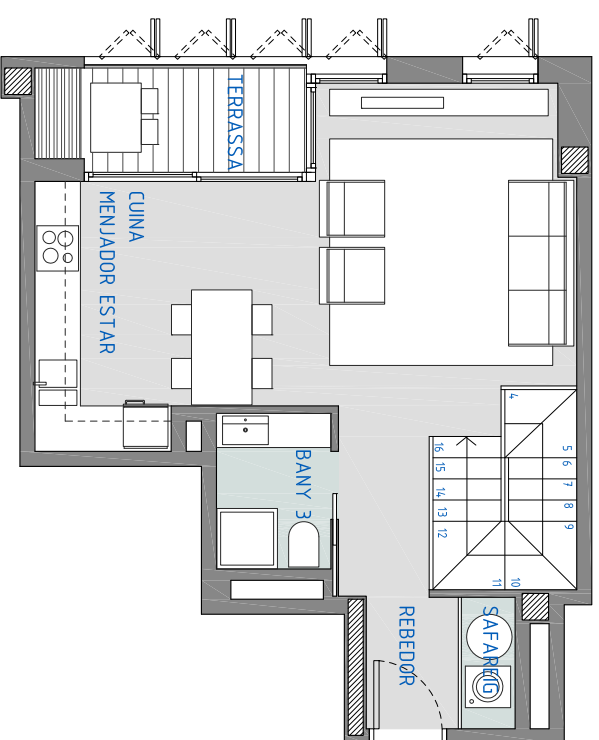
PLANTA SEGONA
