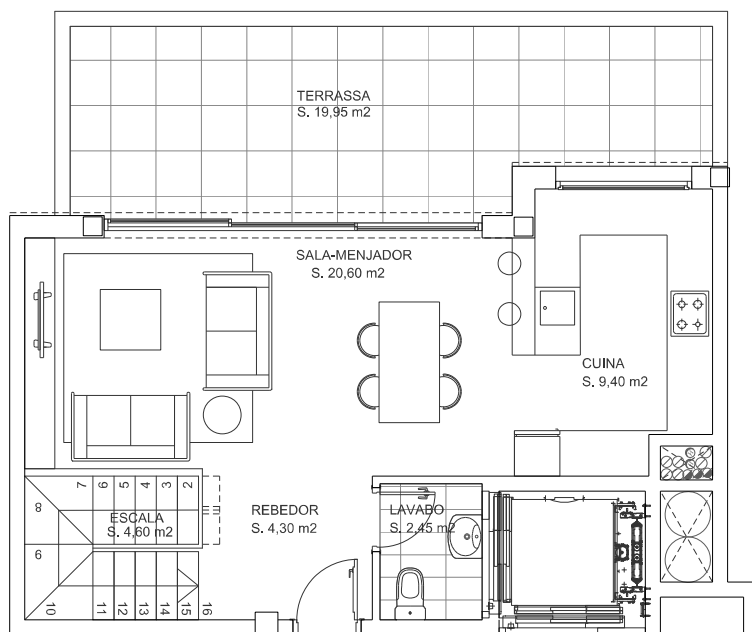
PLANTA PIS SOTACOBERTA
