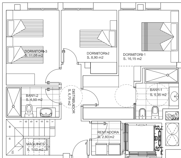
PLANTA PIS SEGON
