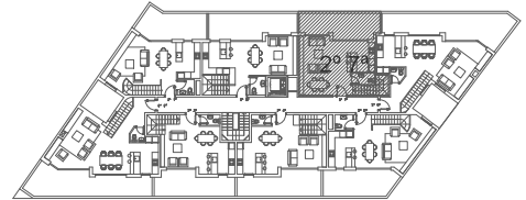
PLANTA SOTACOBERTA
