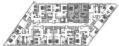
PLANTA SEGONA
