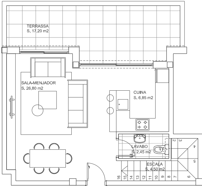
PLANTA SOTACOBERTA
