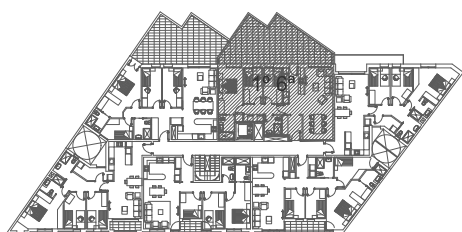
PLANTA PRIMERA
