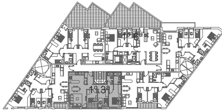
PLANTA PRIMERA
