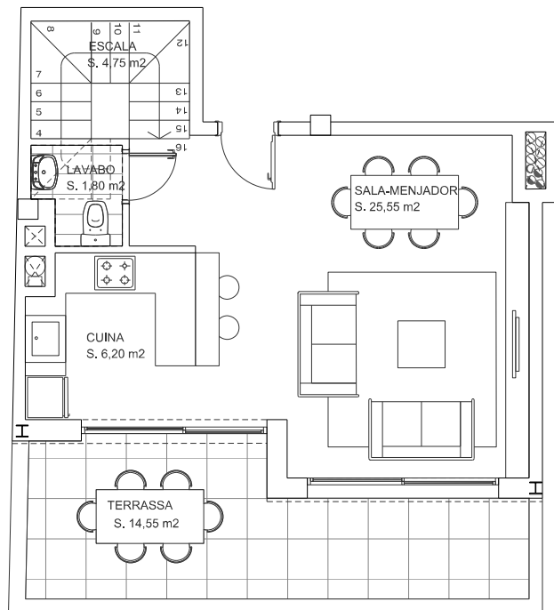
P. SOTACOBERTA 2º 2ª
