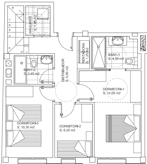
PLANTA PIS 2º 2ª
