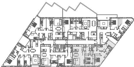
PLANTA PRIMERA
